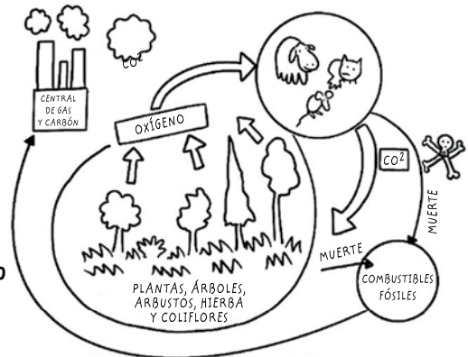
MI ESQUEMA DEL CICLO DEL CARBONO
